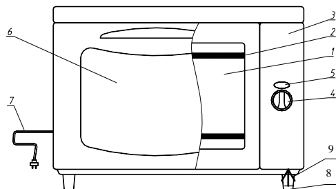
Рис. Б.1 – Устройство электрошкафа
